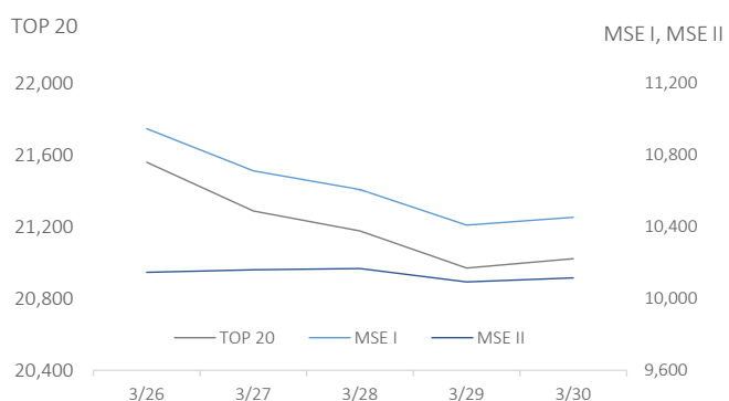
MSE Индекс
